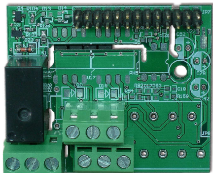
標準型 I/O 擴充卡 (選購配件 A) (內含 FWD/REV/MI1/MI2/DCM/E/R1A/R1B/R1C 端子)
