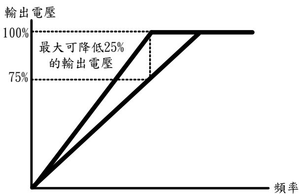
自動省電運行
