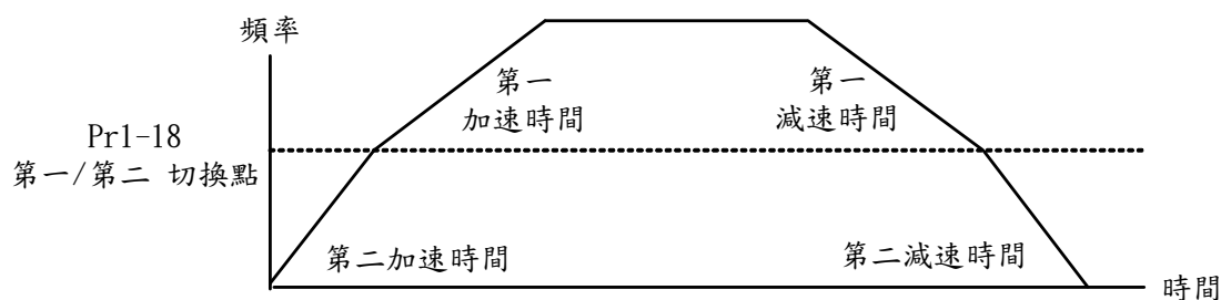
第一/第二 加/減速時間切換
