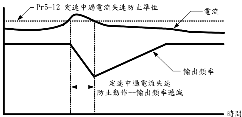
定速中過電流失速防止功能
