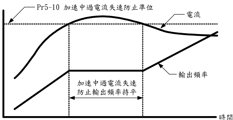
加速中過電流失速防止功能
