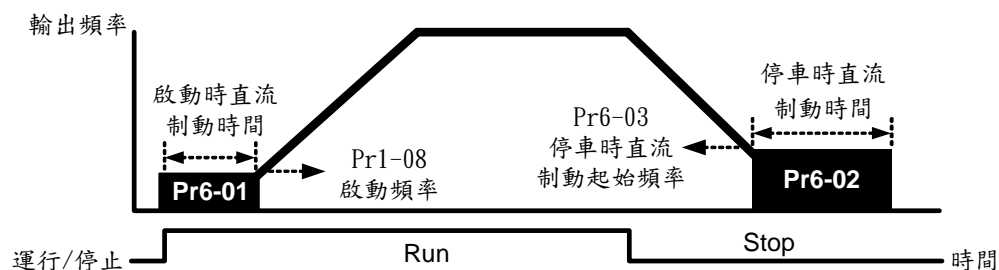
直流制動執行時序圖
