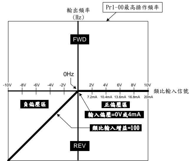
正負偏壓模式為高於偏壓=偏壓 (Pr3-05=2或Pr3-09=2或Pr3-14=2)
