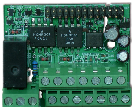
全配型 I/O 擴充卡 (選購配件 C) (內含 FWD/REV/MI1/MI2/MI3/MI4/ DCM/E/+12V/AVI/ACI/DCM/ R1A/R1B/R1C/M01/MCM/AVO 端子)
