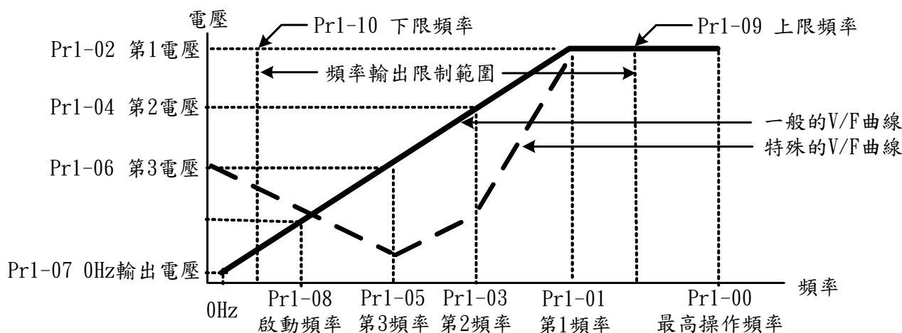
V/F曲線相關參數圖
