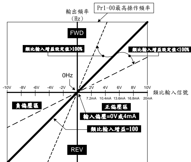
正負偏壓模式為以偏壓為中心 (Pr3-05=0或Pr3-09=0或Pr3-14=0)
