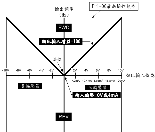
正負偏壓模式為以偏壓為中心取絕對值 (Pr3-05=3或Pr3-09=3或Pr3-14=3)
