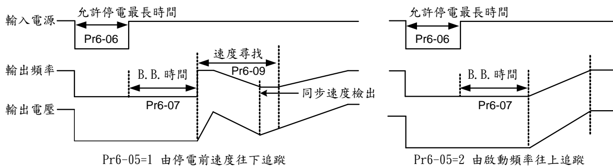
瞬時停電再起動時序圖
