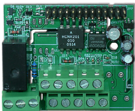
加配型 I/O 擴充卡 (選購配件 B) (內含 FWD/REV/MI1/MI2/MI3/DCM/E/ +12V/AVI/DCM/R1A/R1B/R1C/AVO 端子)
