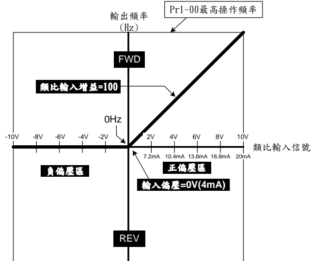
正負偏壓模式為低於偏壓=偏壓 (Pr3-05=1或Pr3-09=1或Pr3-14=1)
